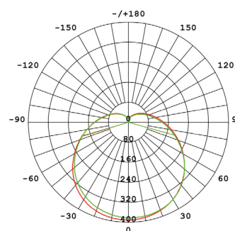
CURVA FOTOMETRICA
